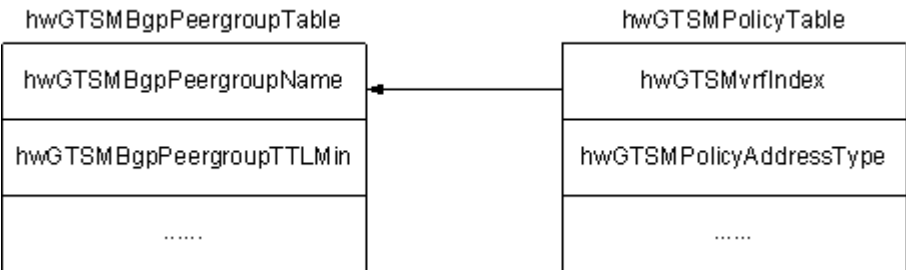
图 54-1 GTSM 策略表的表间关系图
