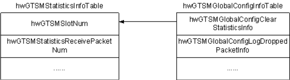
图 54-2 GTSM 报文统计表与全局配置表的关系图
